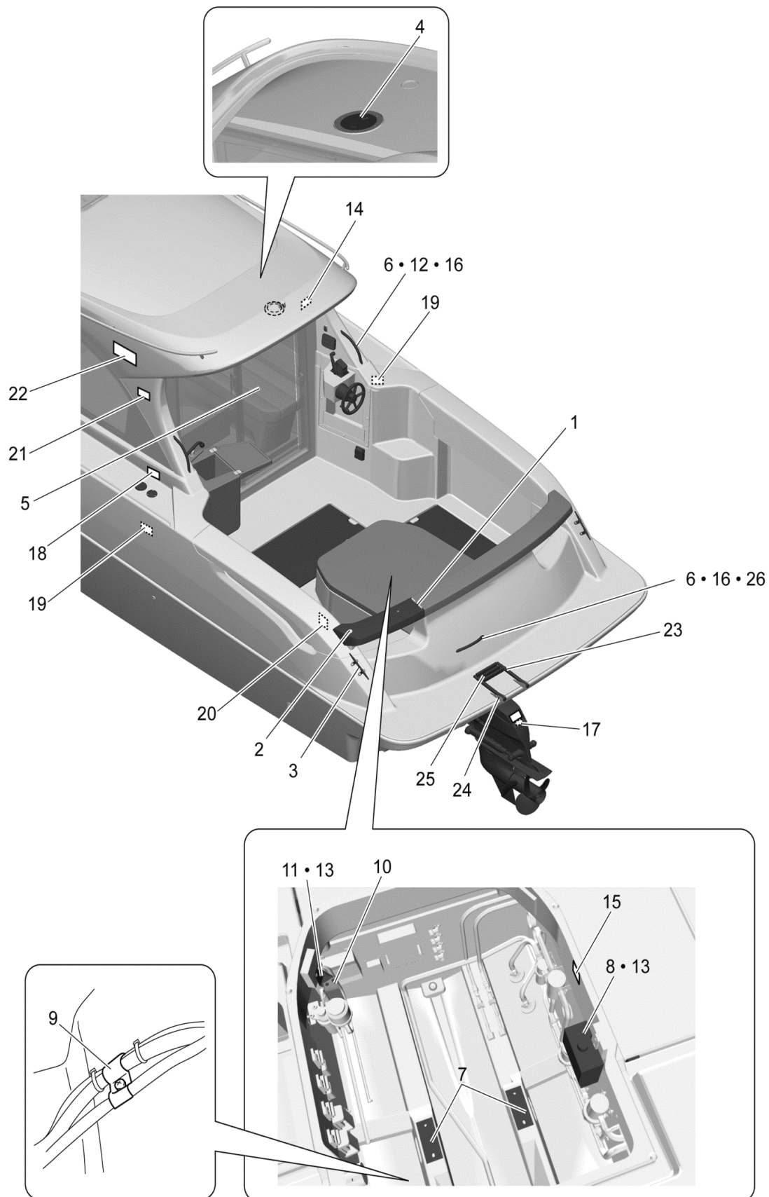
Fig. 4 アフトデッキ(2)
