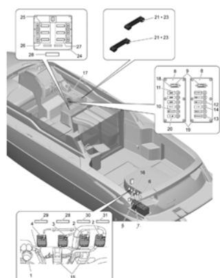
Fig.22 電源装置
