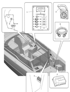
Fig.23 AC電源(オプション)
