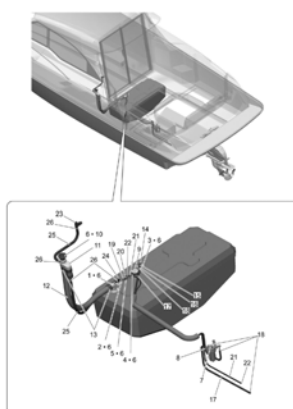
Fig.17 フューエルライン ..... P.34
