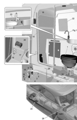
Fig.9 マリントイレ(1)(オプション) ..... P.18
