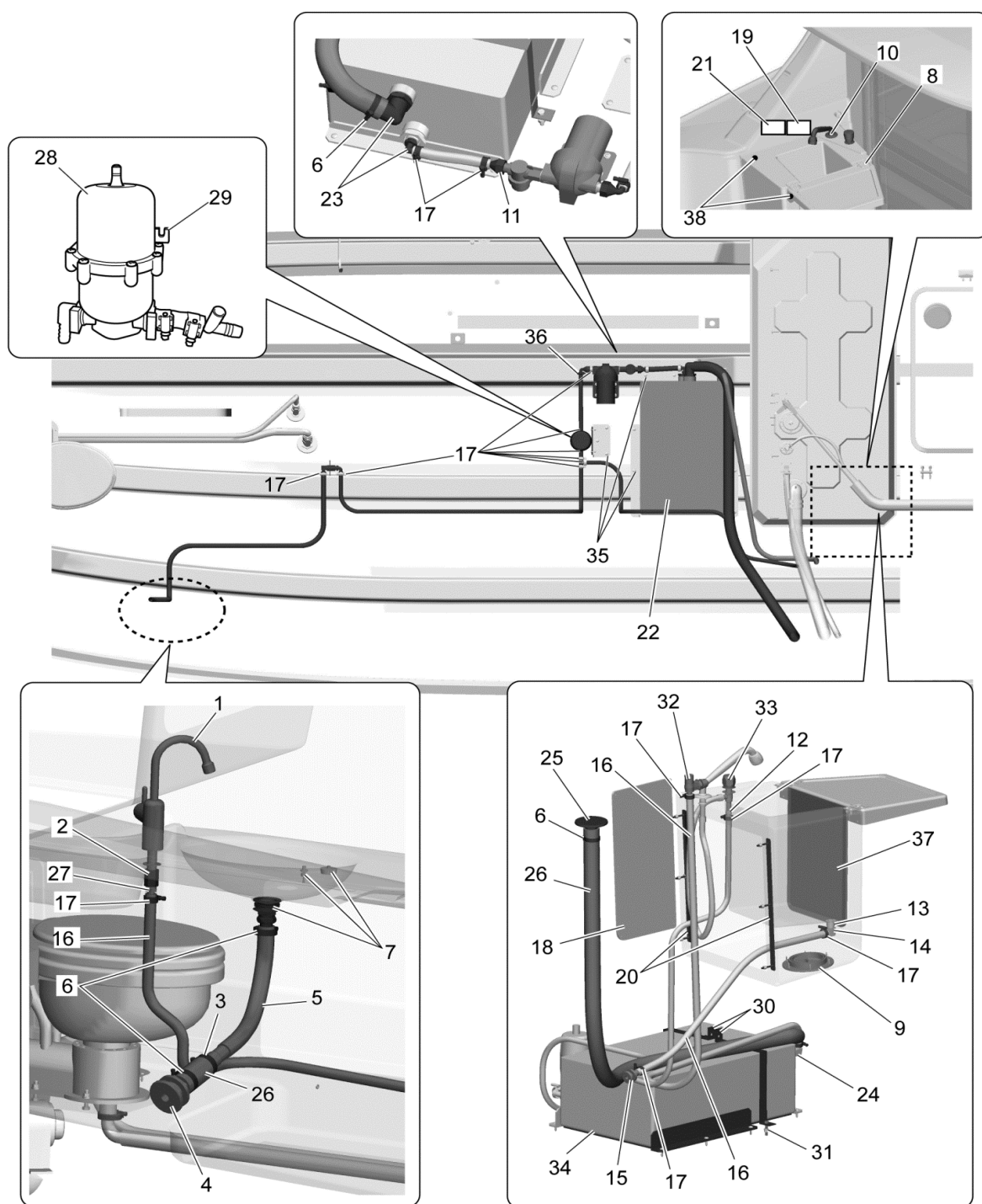
Fig. 11 清水システム(1)(オプション)
