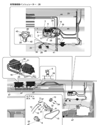
Fig.19 エアコン (2)(オプション)
