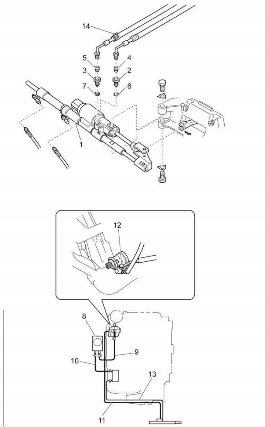
Fig. 15 パワーステアリング
