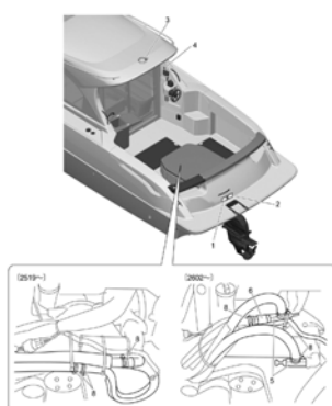
Fig.5 アフトデッキ(3) ..... P.10
