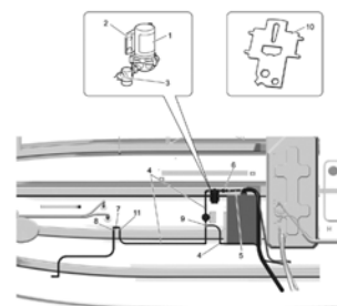
Fig.12 清水システム(2)(オプション) ..... P.24
