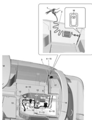
Fig.13 デッキウォッシュシステム(オプション) ..... P.26
