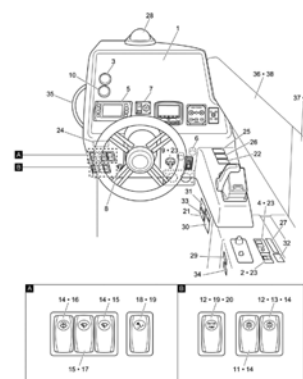
Fig.6 ロアヘルムメーターパネル ..... P.12
