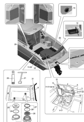
Fig.3 アフトデッキ(1) ..... P.6
