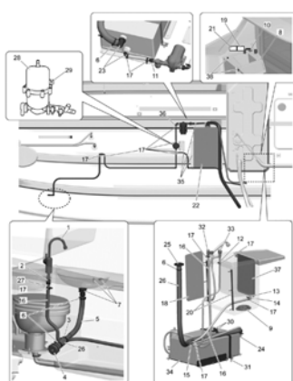
Fig.11 清水システム(1)(オプション) ..... P.22
