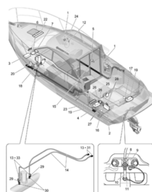
Fig.21 ハウスラスター・トヨタハ・チャルアンカー システム(オプション)..... P.42
