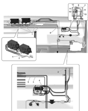
Fig.20 エアコン (3)(オプション)
