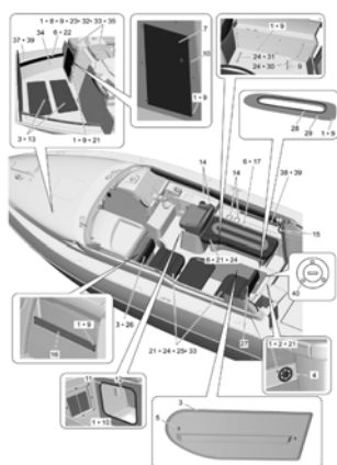
Fig.7 室内 装備品(1) ..... P.14
