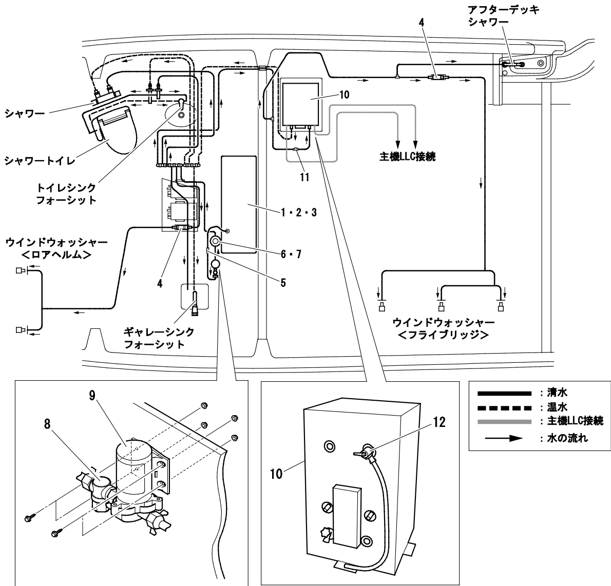
Fig. 9 清水システム
