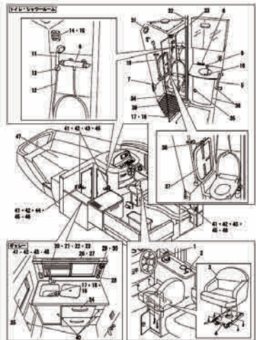
Fig.6 室内 装備品
