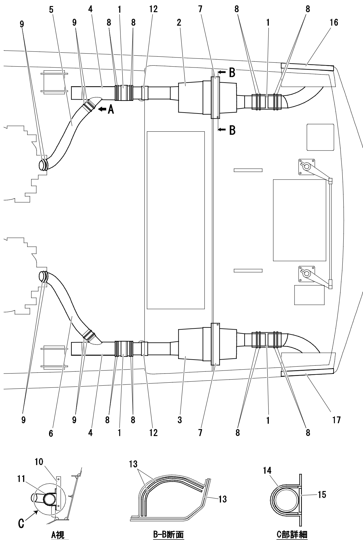
Fig. 22 エキゾースト
