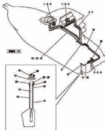
Fig.18 ステアリング ..... P.34
