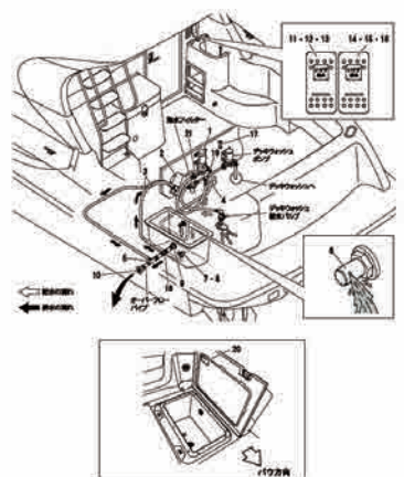
Fig.25 いけす ..... P.46
