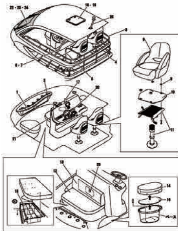
Fig.6 室内 装備品
