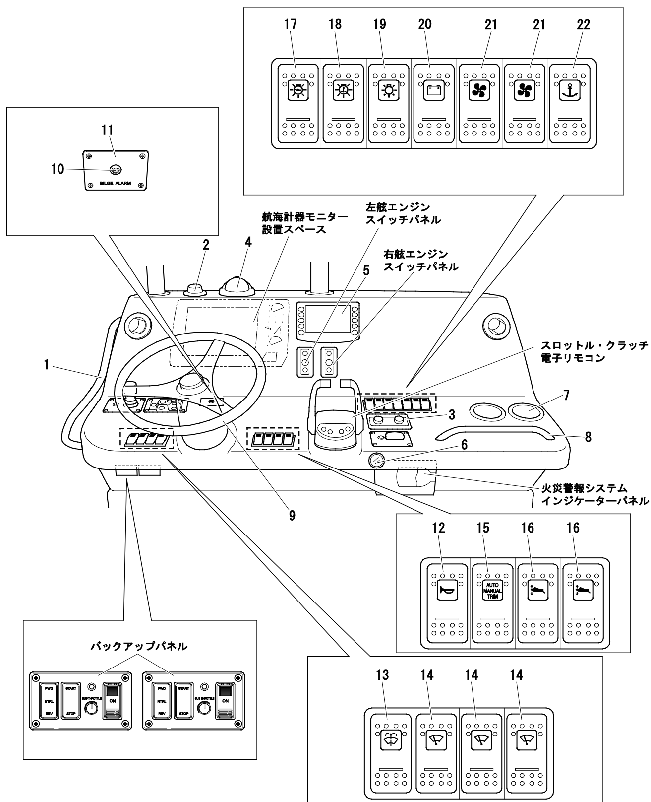
Fig. 5 フライブリッジメーターパネル
