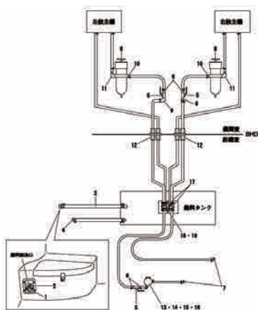
Fig.15 フューエルライン
