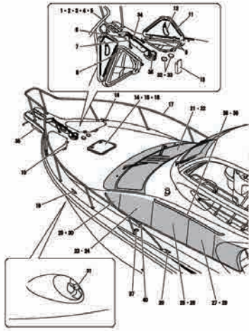
Fig.3 フライブリッジ
