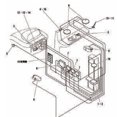
Fig.17-1 オーディオ&ジョイフルトーク
