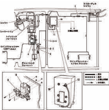
Fig.9 清水システム
