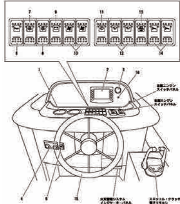
Fig.4 ロアヘルムメーターパネル
