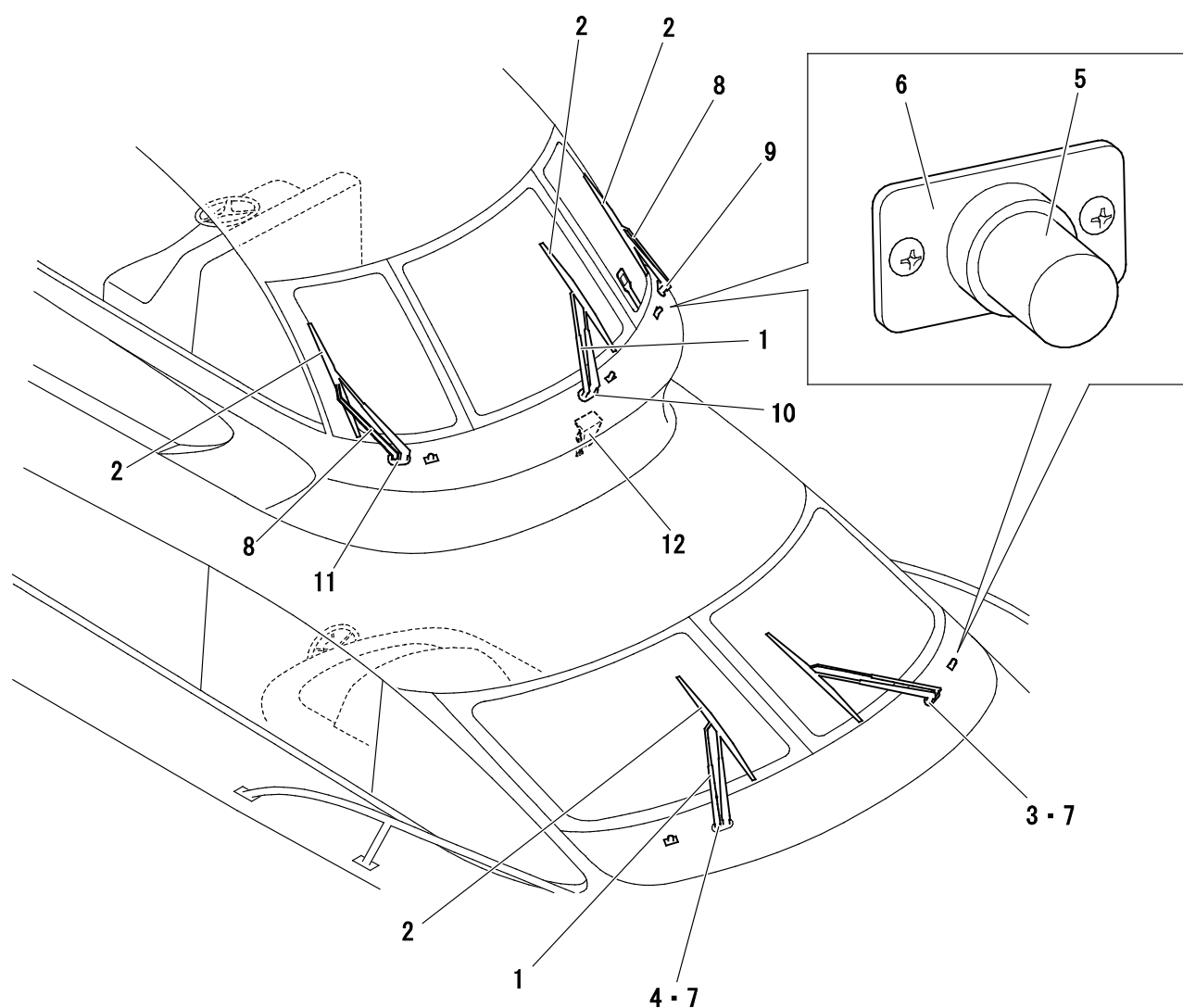
Fig. 8 ワイパー&amp;ホーン
