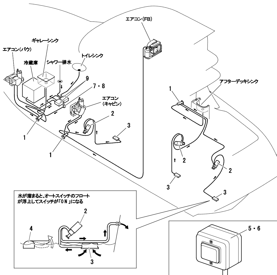
Fig. 11 ビルジポンプ
