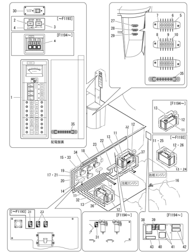
Fig.30 電源装置 & ワイヤハーネス ..... P.52
