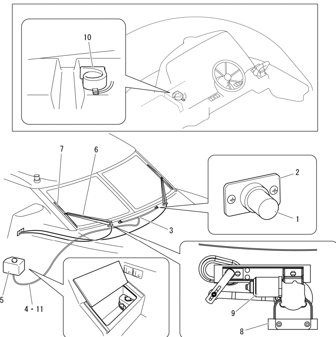
Fig. 11 ワイパー&amp;ホーン
