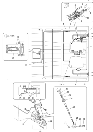
Fig.27 オートフラップ(オプション)(油圧式) ..... P.46
