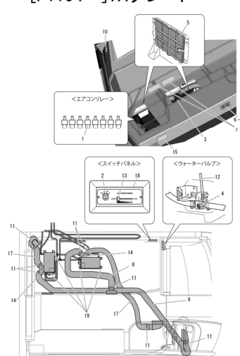
Fig.24 陸電式エアコン(オプション) ..... P.41
