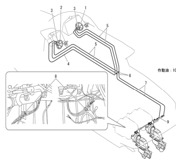
Fig.15 マニュアルステアリング
