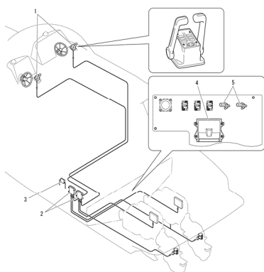
Fig. 10 電子リモコン
