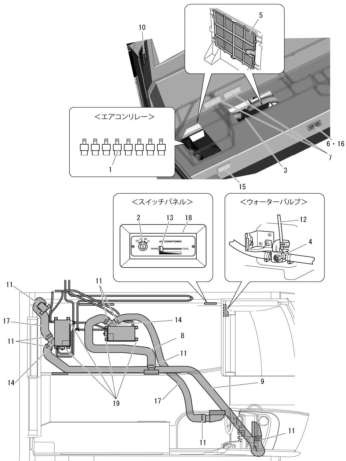
Fig. 21 主機駆動式エアコン(室内部品)[F1194~]:Xグレード
