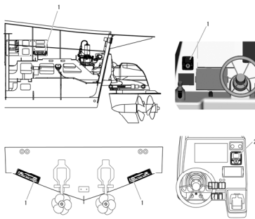
Fig.28 オートフラップ(オプション)(電動式) ..... P.48
