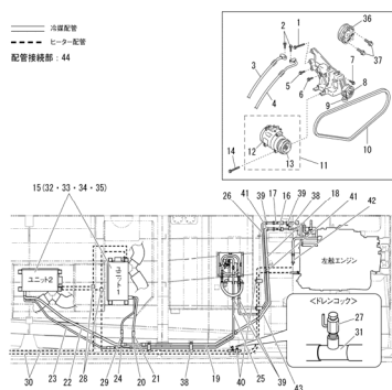
Fig.22 主機駆動式エアコン(室外部品) (1) ..... P.38
