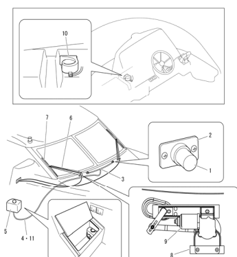
Fig. 11 ワイパー&ホーン
