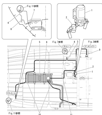
Fig. 13 清水システム
