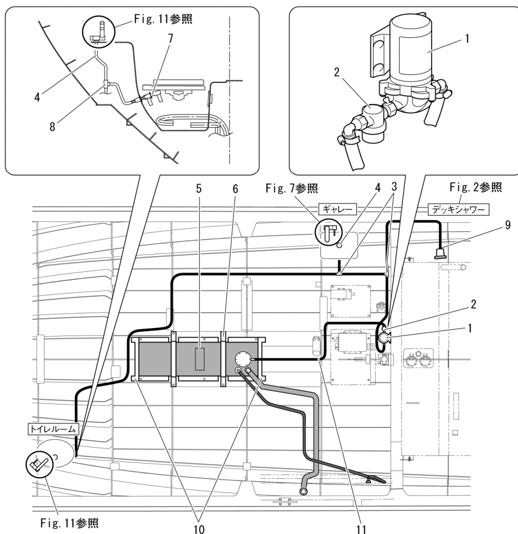
Fig. 13 清水システム
