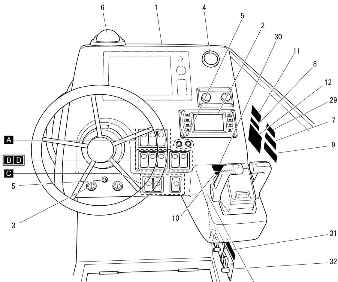
Fig. 6 ロアヘルムメーターパネル
