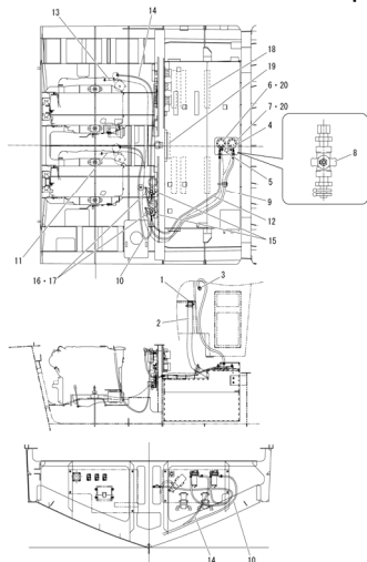
Fig.22 主機駆動式エアコン(室外部品) (1) ..... P.38
