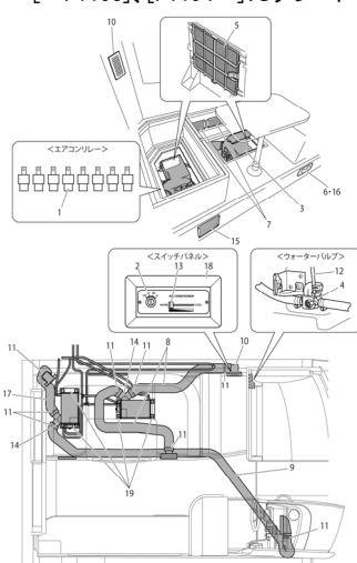
Fig.23 主機駆動式エアコン(室外部品) (2) ..... P.40
