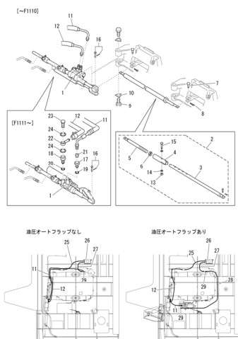
Fig.16 パワーステアリング
