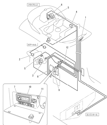
Fig.25 オーディオ&ジョイフルトーク (オプション)..... P.42
