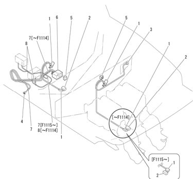
Fig.17 ビルジポンプ
