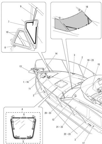
Fig.4 フライブリッジ
