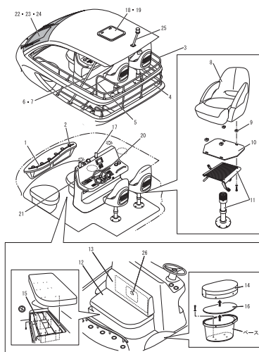
Fig.6 室内 装備品
