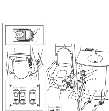
Fig.7 マリントイレ
