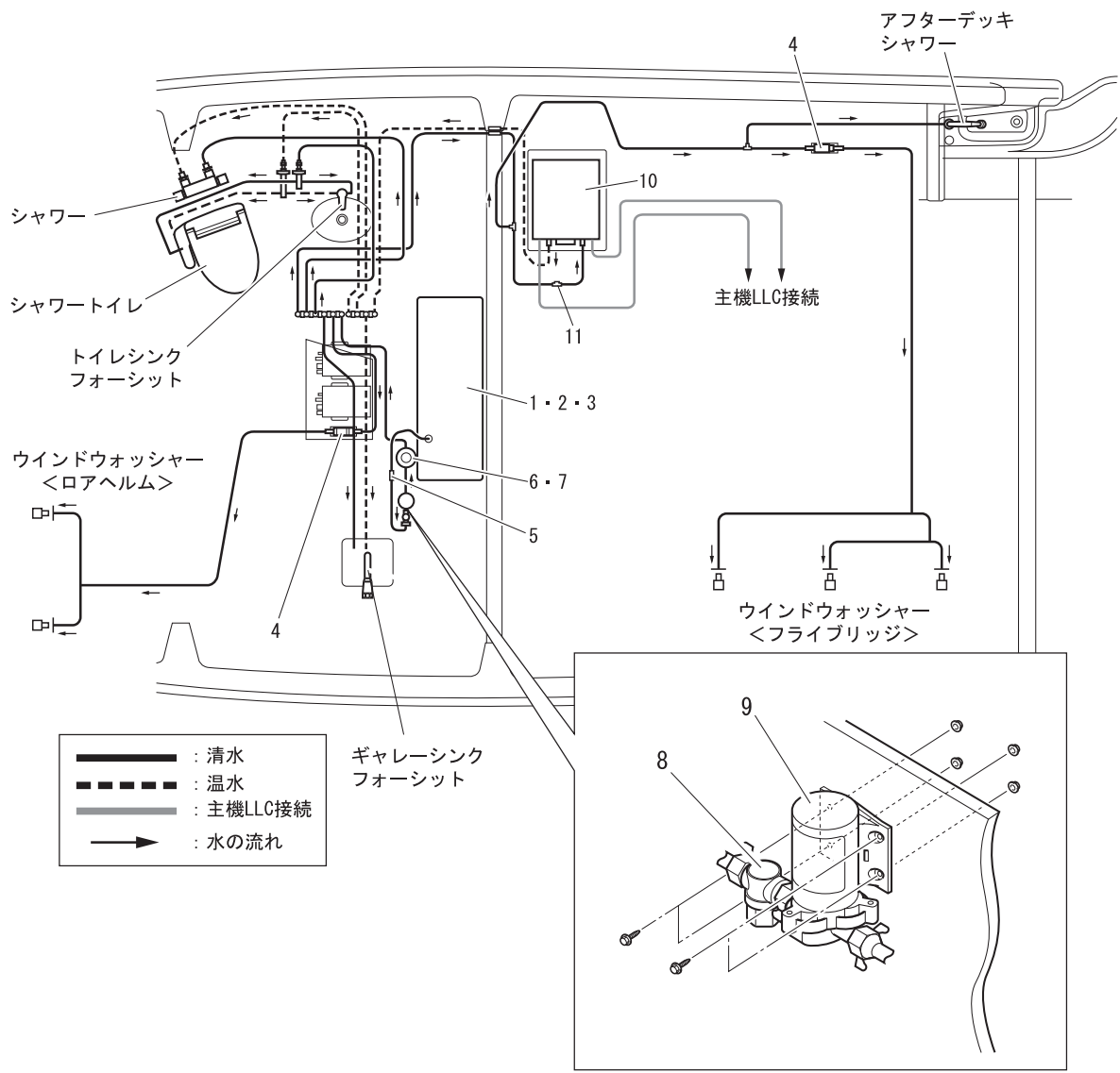
Fig. 9 清水システム
