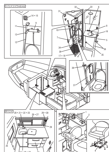
Fig.6 室内 装備品
